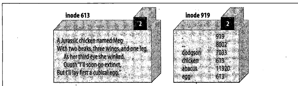
图13-2: egg被链接到chicken
