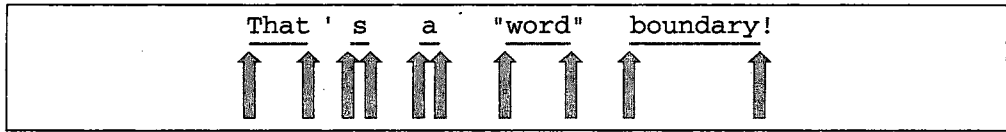
图8-1：用\b匹配单词边界
