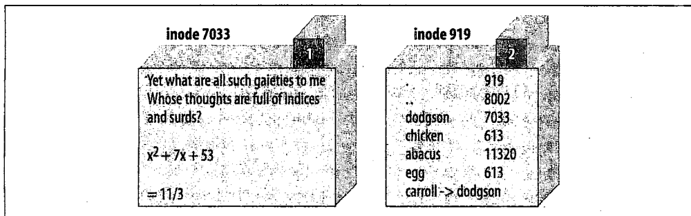
图13-3：指向inode7033的符号链接
