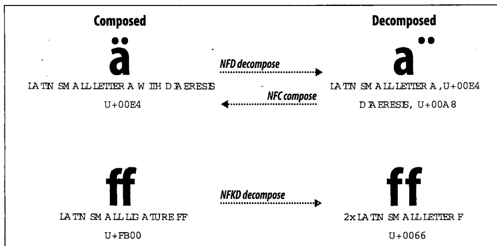
图C-2: 我们可以分解并重新组合完全等价的字素表示形式, 但只能分解不完全等价的字素表示形式。
