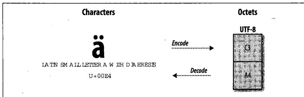
图C-1：代码点只是字符代号，并非存储内容。编码就是把字符转换为存储位组的过程。
