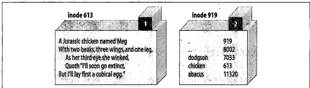
图13-1：先有chicken再有egg
